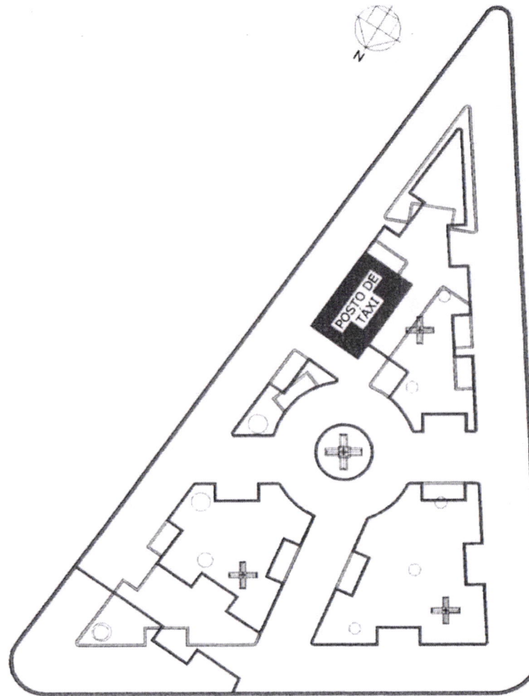
PLANTA BAIXA - REFORMA 1:75
