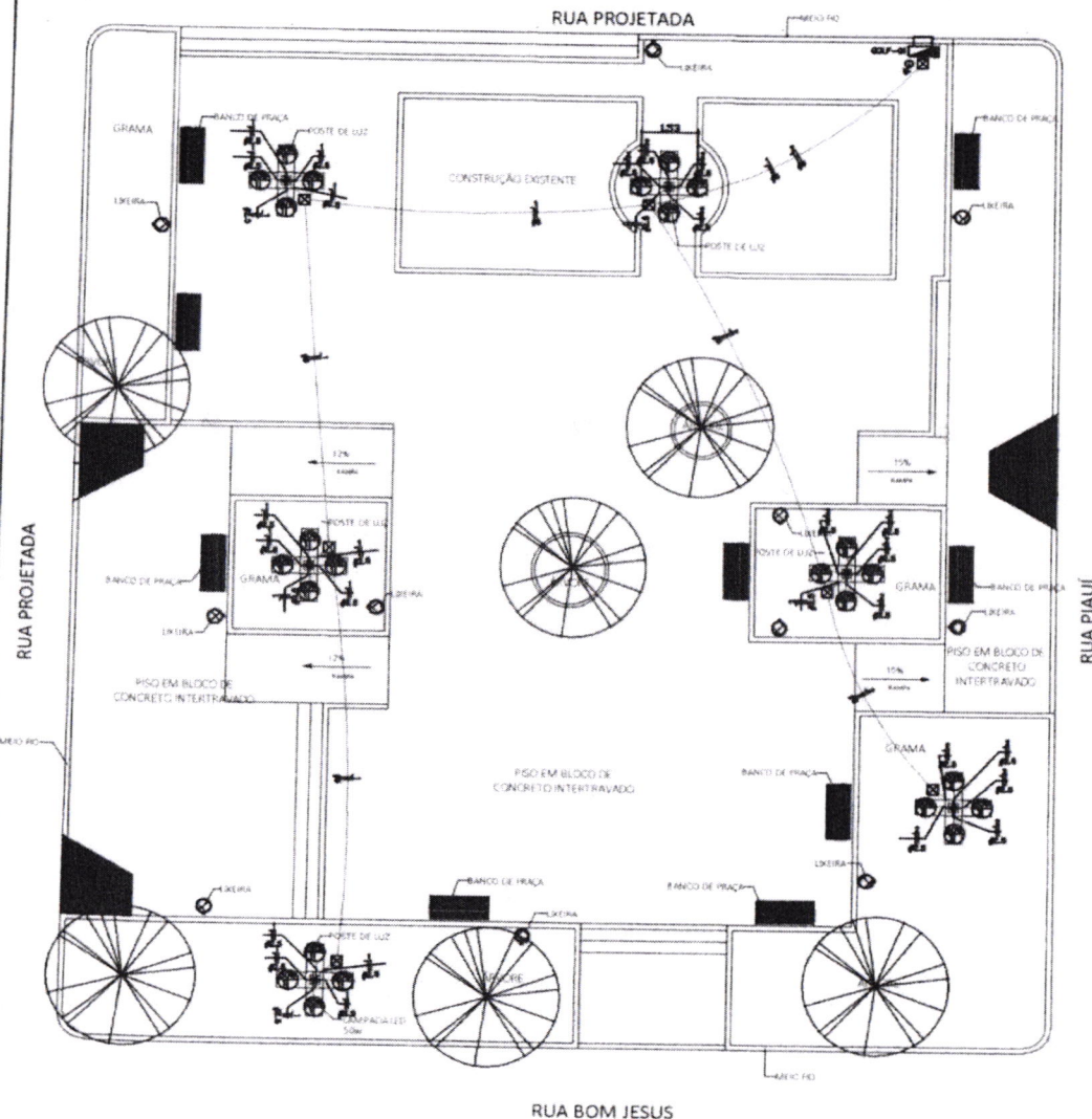
PLANTA BARRA - ILUMINAÇÃO
