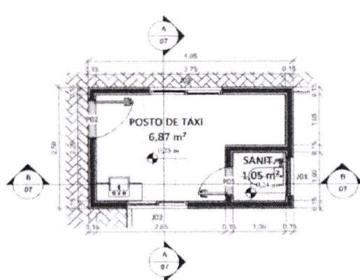
PLANTA BAIXA - POSTO 1 : 50
