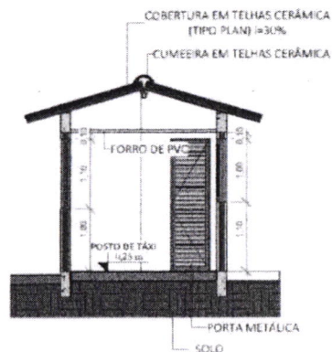
CORTE AA 1 : 50
