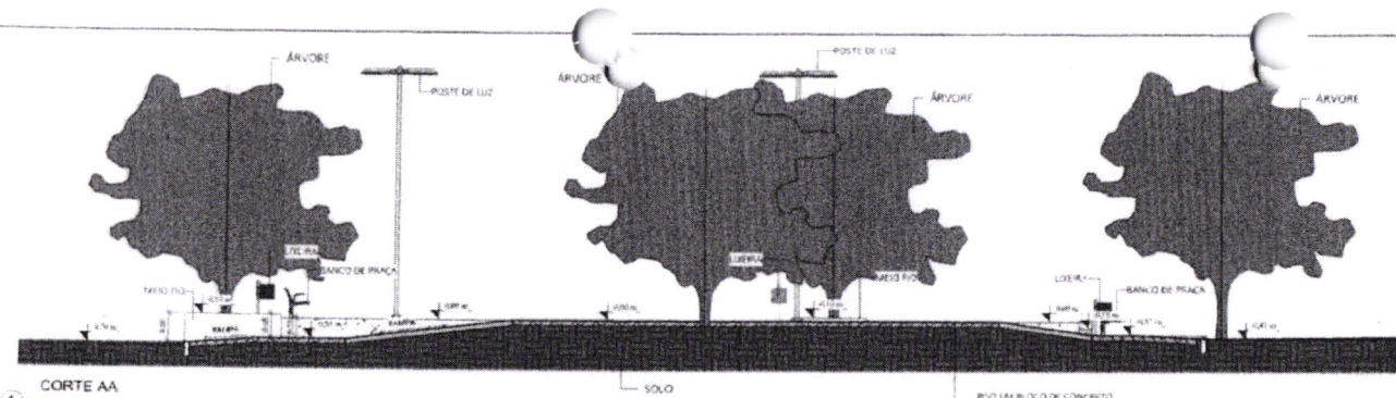
1 CORTE AA 1 : 75
