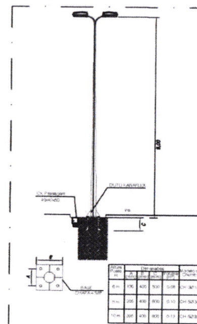
DETALHE "C" POSTE RETO S/ESC
