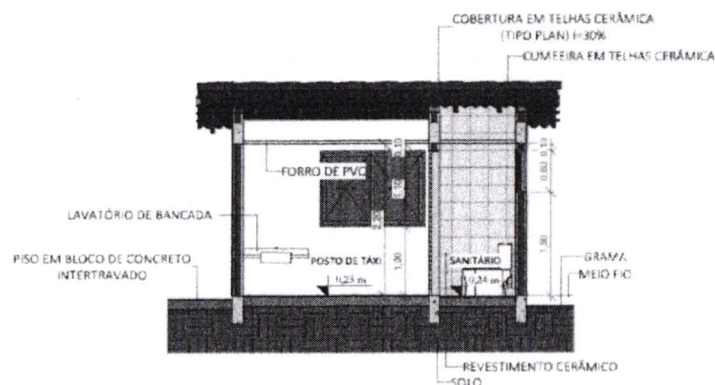
CORTE BB 1 : 50
