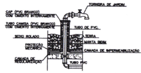
DETALHE TORNEIRA DE JARDIM SEM ESCALA
