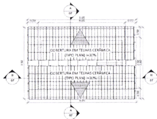
PLANTA DE COBERTURA - POSTO 1 : 50
