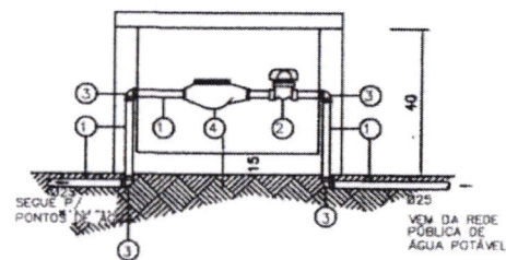
DETALHE 01 HIDROMETRO SEM ESCALA
