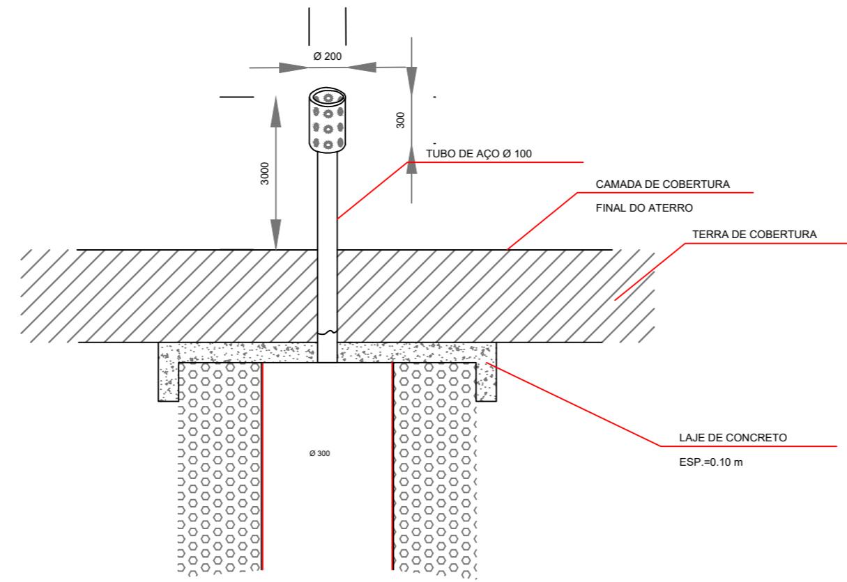
DETALHE DE UM QUEIMADOR DE GÁS (FLAIR) S/ESCALA
