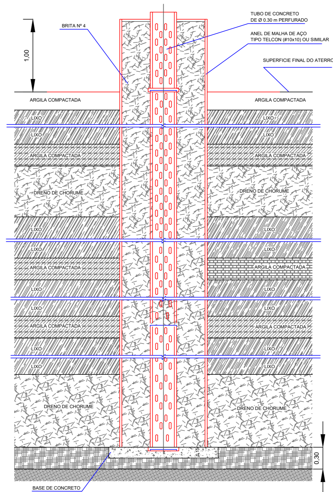
CORTE AA ESCALA 1:25
