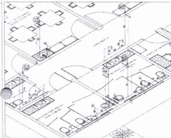
ISOMETRICO 1:25
