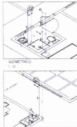
ISOMETRICO 1:25
