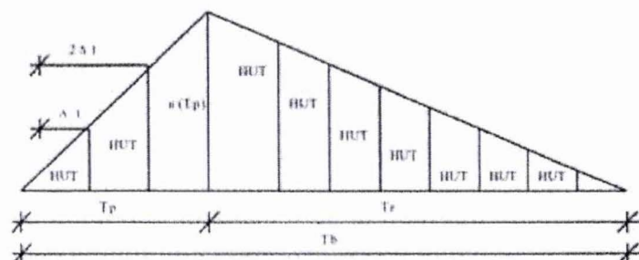
Figura 10 – Hidrograma Unitário Triangular
