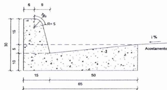
Seção transversal
