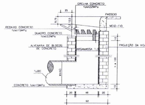
CORTE BB'
