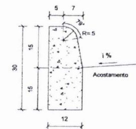
Seção transversal
