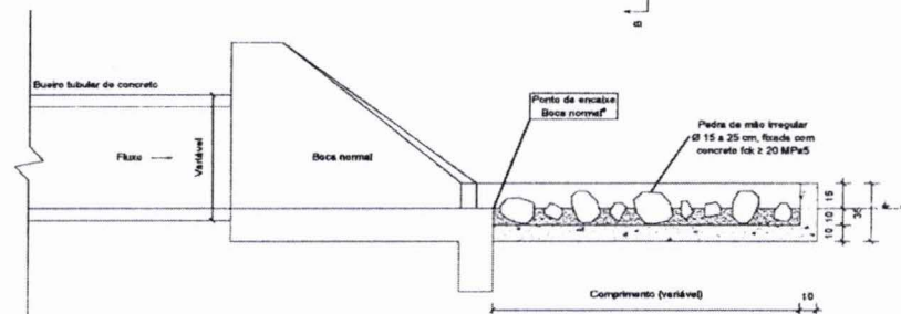
Corte A-A' Sem escala
