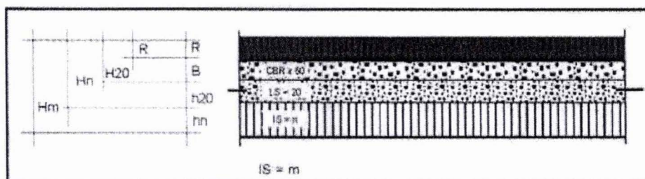
Figura 4 – Nomenclatura de camadas no dimensionamento do pavimento
