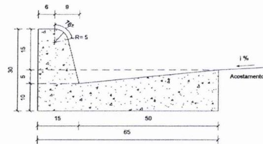
Seção transversal
