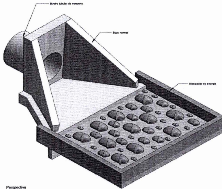
Perspectiva
