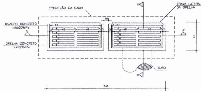
PLANTA
