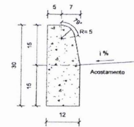
Seção transversal
