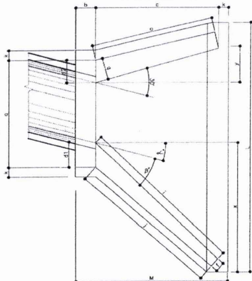
PLANTA ESCONÇO
