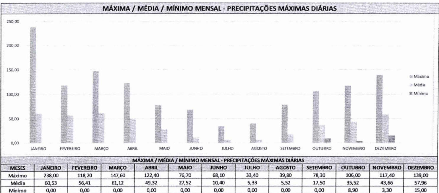
Figura 1 – Precipitação Máxima, Média e Mínima – Precipitações máximas diárias
