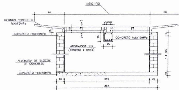
CORTE AA'
