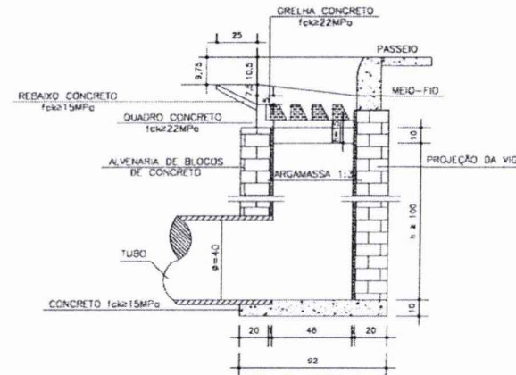
CORTE BB'
