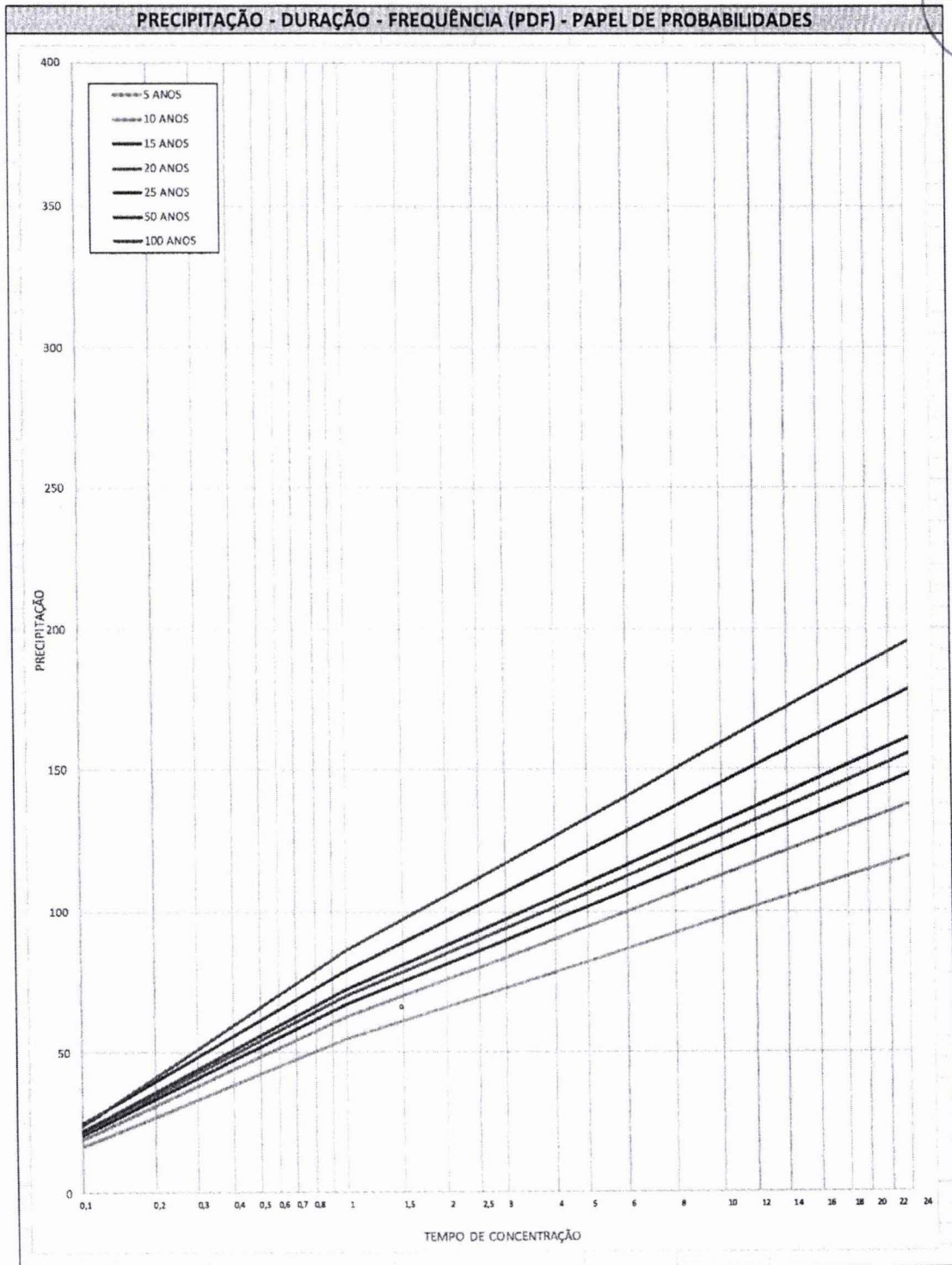
Figura 7 - Papel de Probabilidade – Precipitações por TR
