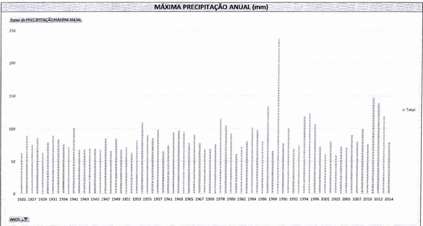
Figura 2 - Total Precipitado (mm/ano)
