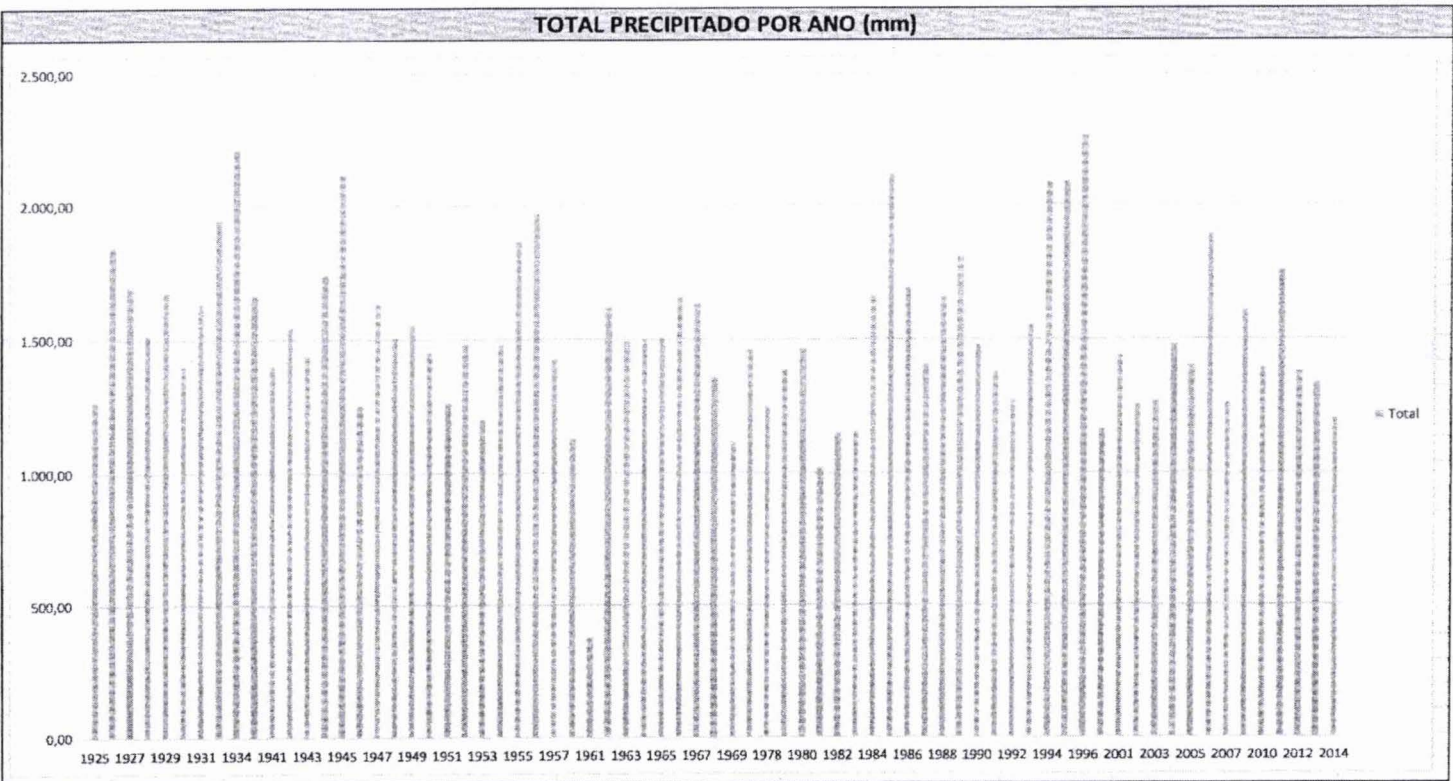
Figura 5 - Total precipitado ao ano (mm)
